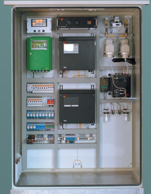
O 2 /CO/NO Betriebsmessung O 2 /CO/NO Process analyser
