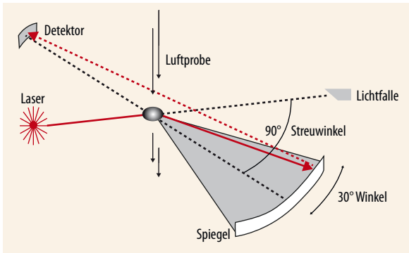
Abb. 2 Bei der optischen Messung von Feinstaubpartikeln passieren diese einzeln einen Laserstrahl. Da die Teilchen abhängig von ihrer Größe gestreut werden, lässt sich aus dem Streuwinkel auf die Partikelgröße schließen.
