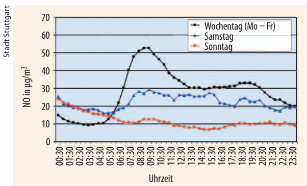
Abb. 1 Im mittleren Tagesgang ist die Konzentration von Stickstoffmonoxid an der Messstation Stuttgart-Mitte besonders hoch im morgendlichen Berufsverkehr.
